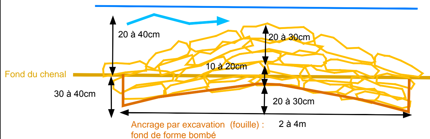
Coupe longitudinale médiane de la rampe en selle de cheval
