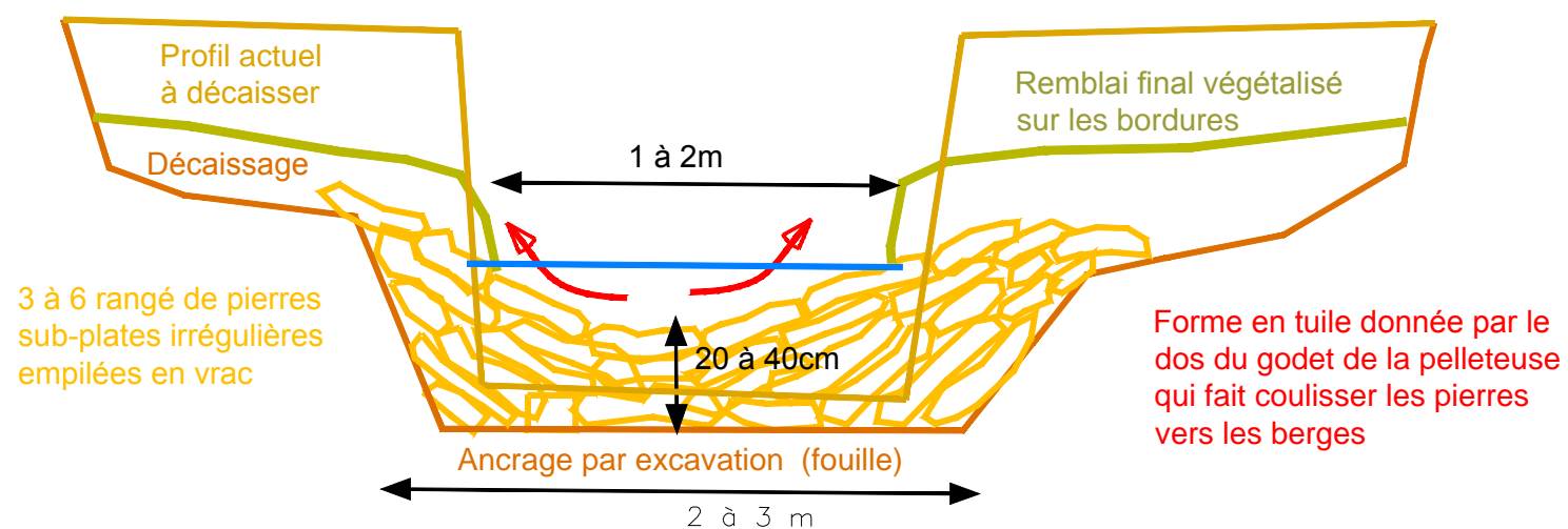
Coupe transversale de la rampe en selle de cheval
