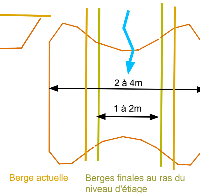
Ancrage vue du haut
